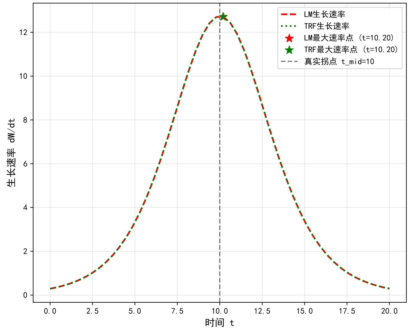
生长速率曲线与最大速率点
