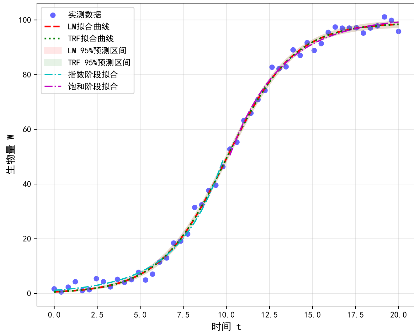
Logistic模型拟合 (含95%预测区间)
