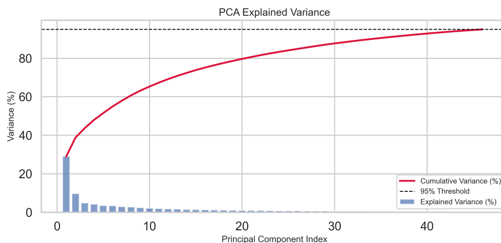
شکل ۱۶: درصد واریانس توضیح داده شده و تجمعی مؤلفه‌های اصلی
