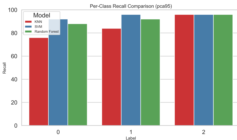
شکل ۲۱: مقایسه Recall هر کلاس بین مدل ها pca95
