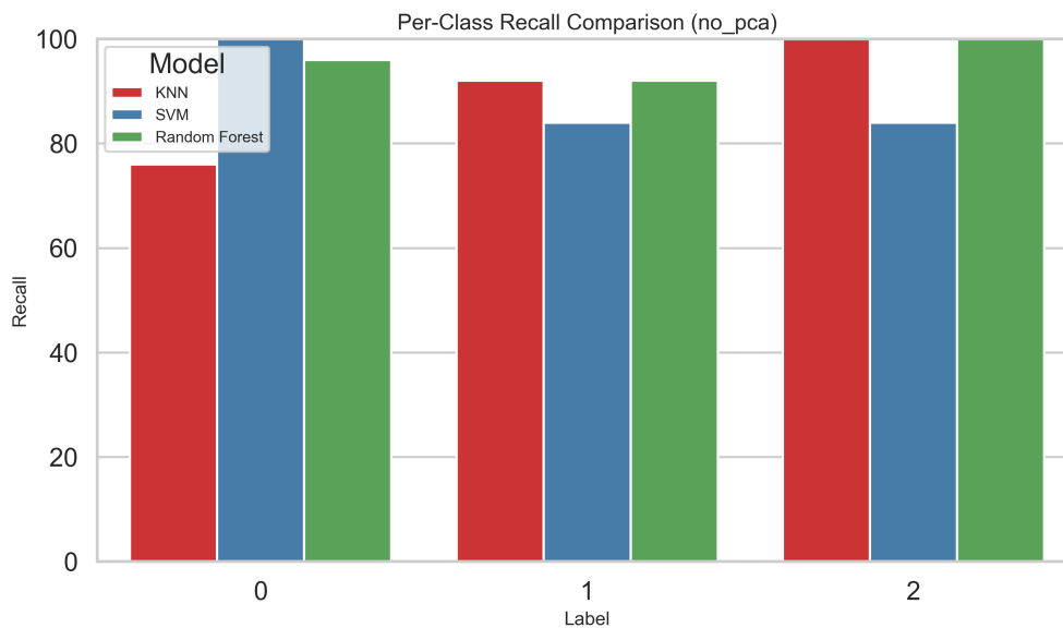
شکل ۲۰: مقایسه Recall هر کلاس بین مدل ها no_pca
