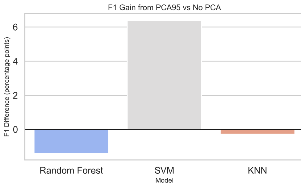
شکل ۱۸: تغییر F1 هر مدل پس از اعمال PCA95
