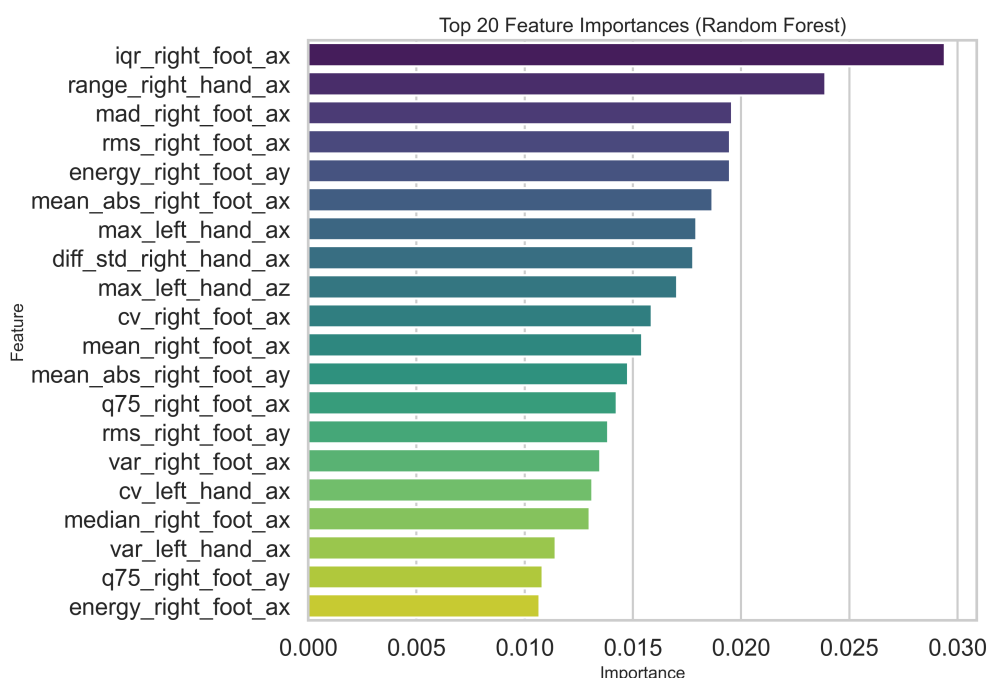
شکل ۱۹: ۲۰ ویژگی برتر بر اساس اهمیت در مدل Random Forest
