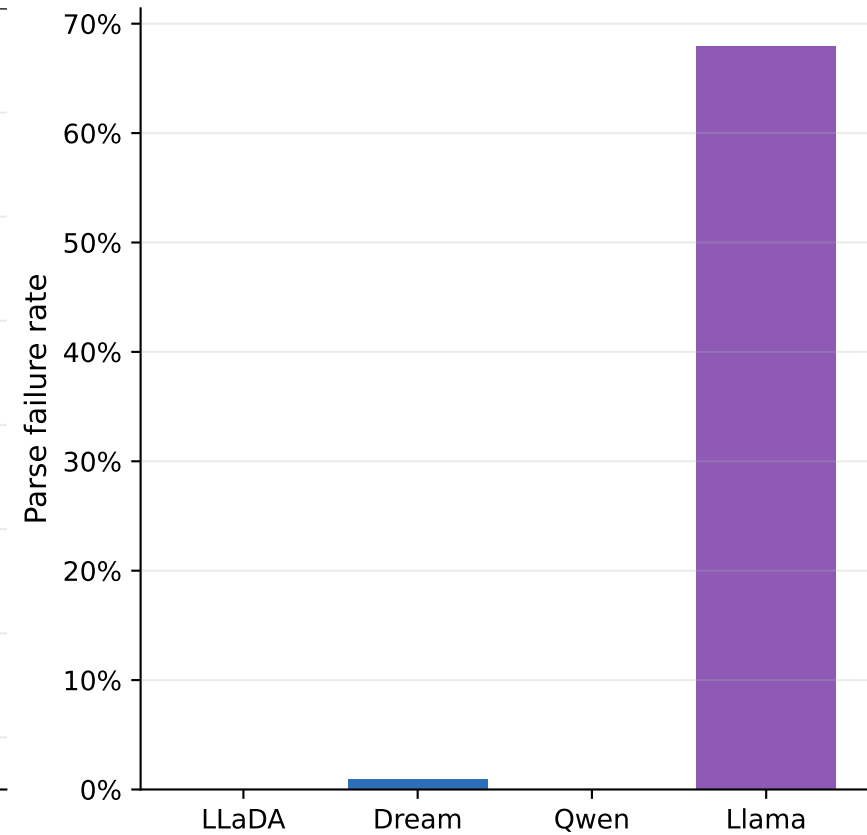
Trip malformed-plan rate
