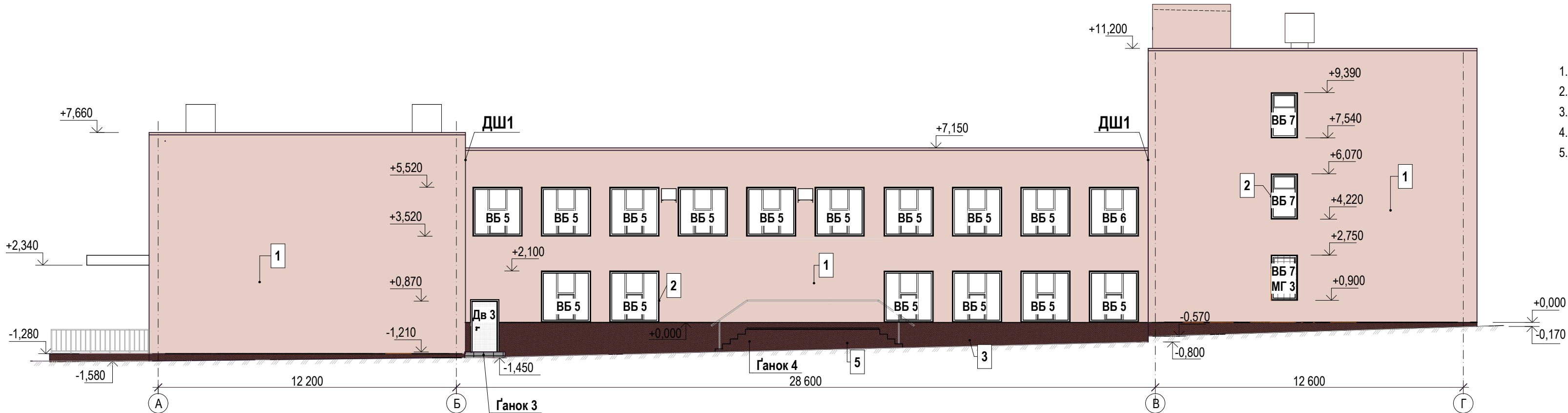
Фасад А-Г
