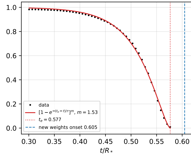
lb0.069_g2
