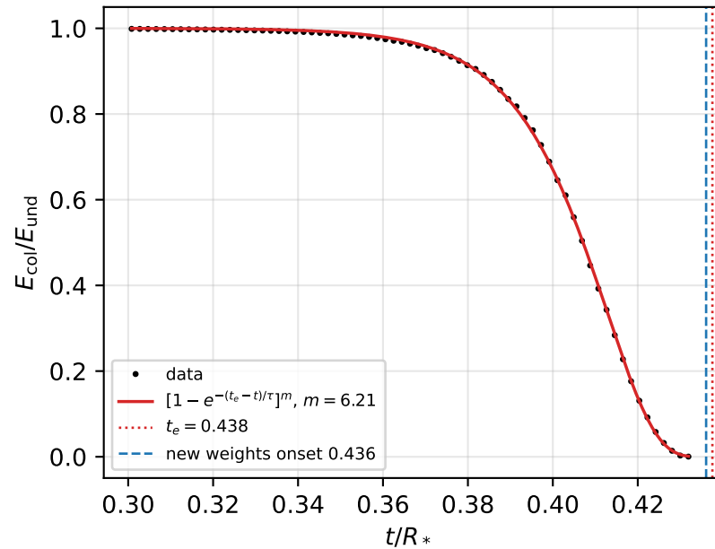
lb0.84_g2
