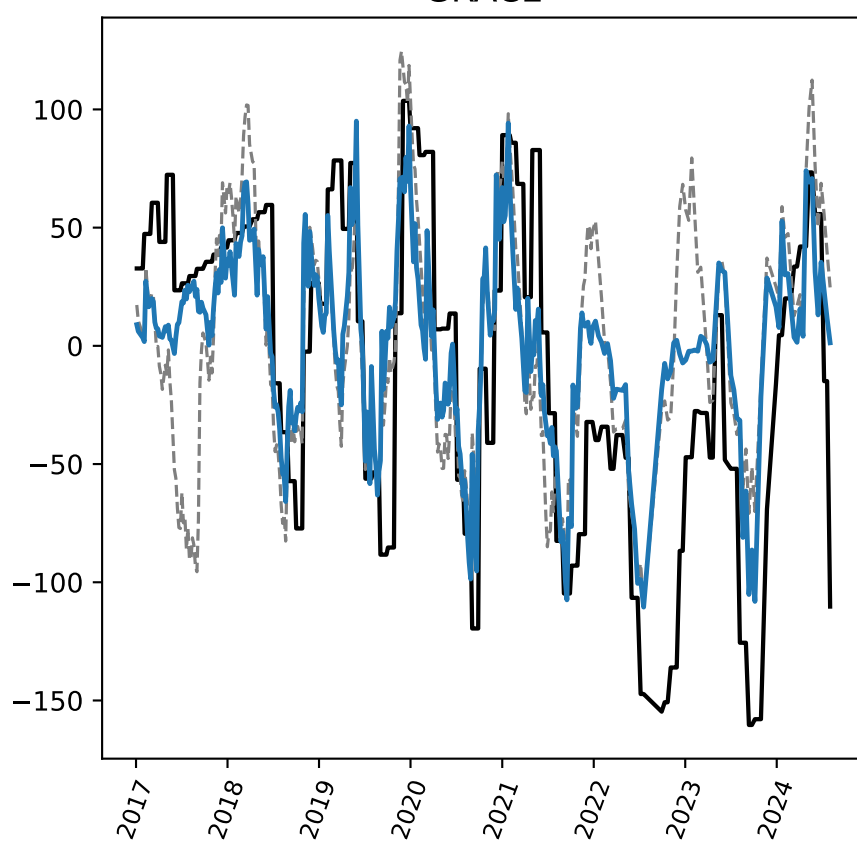
GRACE
