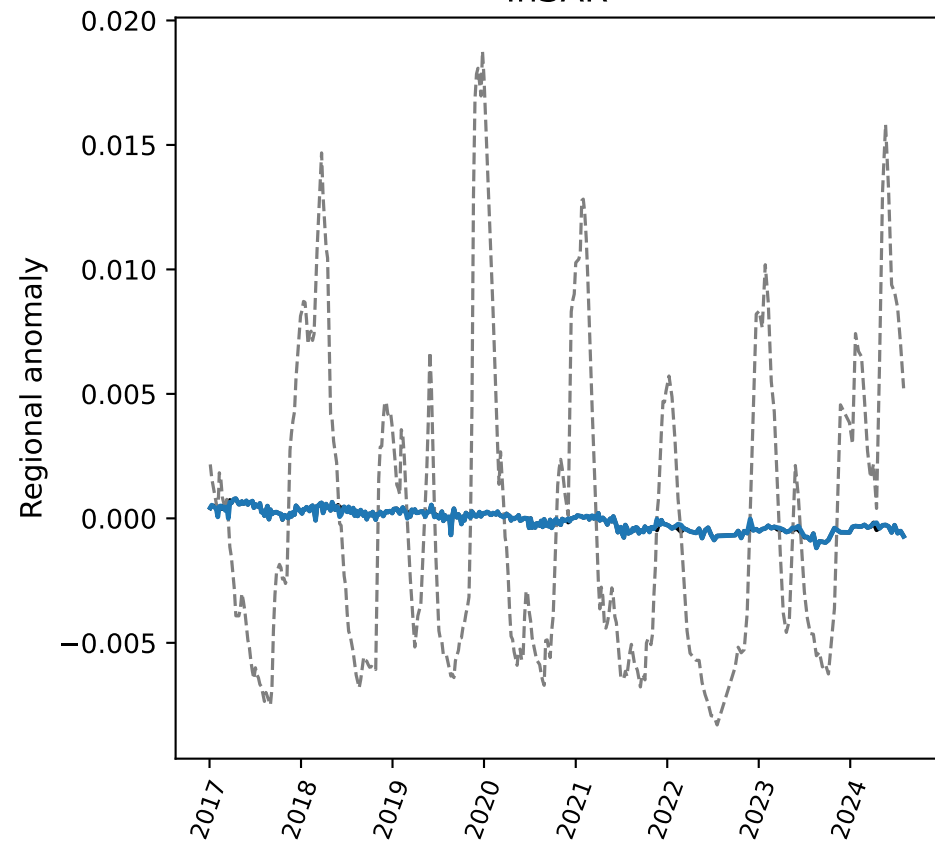
InSAR
