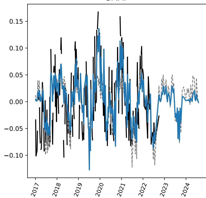
SMAP
