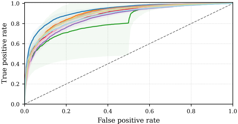
Model (AUC %)
