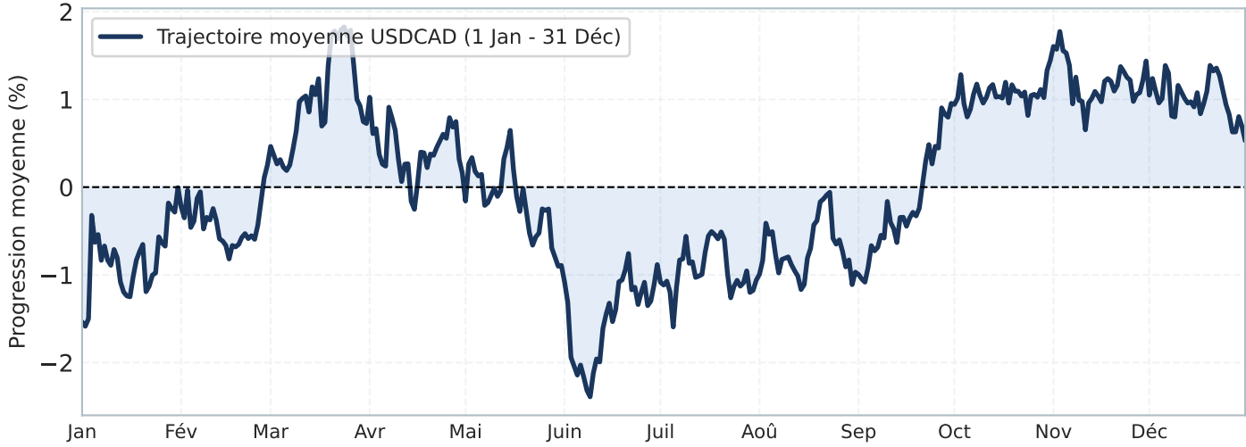
Profil Saisonnier Composite Annuel (Moyenne cumulative sur 365 jours)
