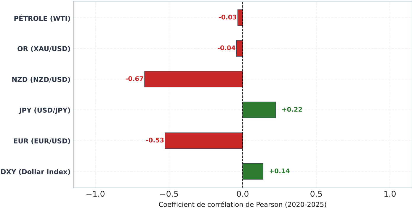
Graphique 5 : Degré de corrélation de USDCAD avec les 6 piliers macro
