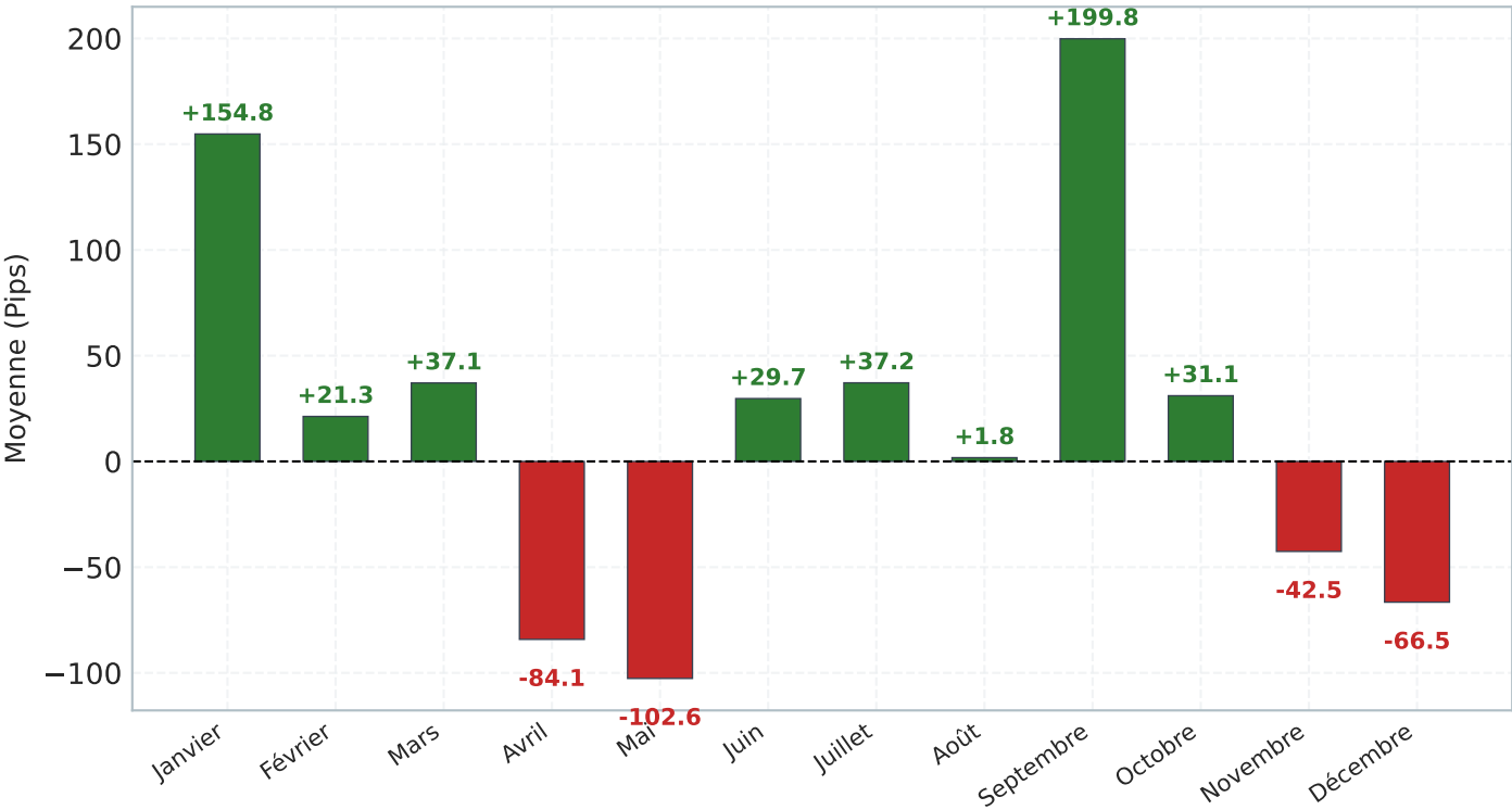
Graphique 1 : Pips moyen par mois (USDCAD)
