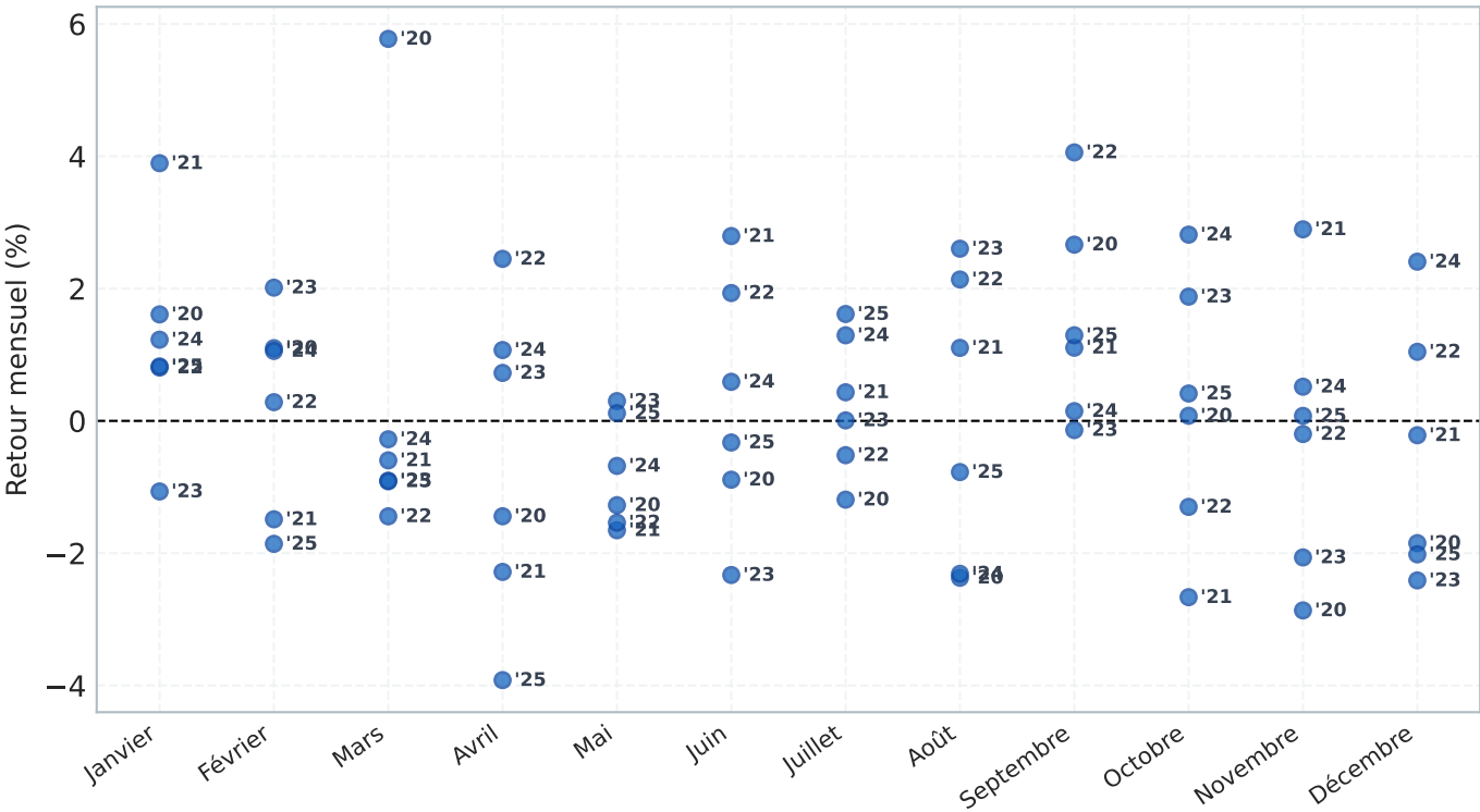
Graphique 2 : Nuage de points des retours mensuels (%) pour USDCAD (2020-2025)
