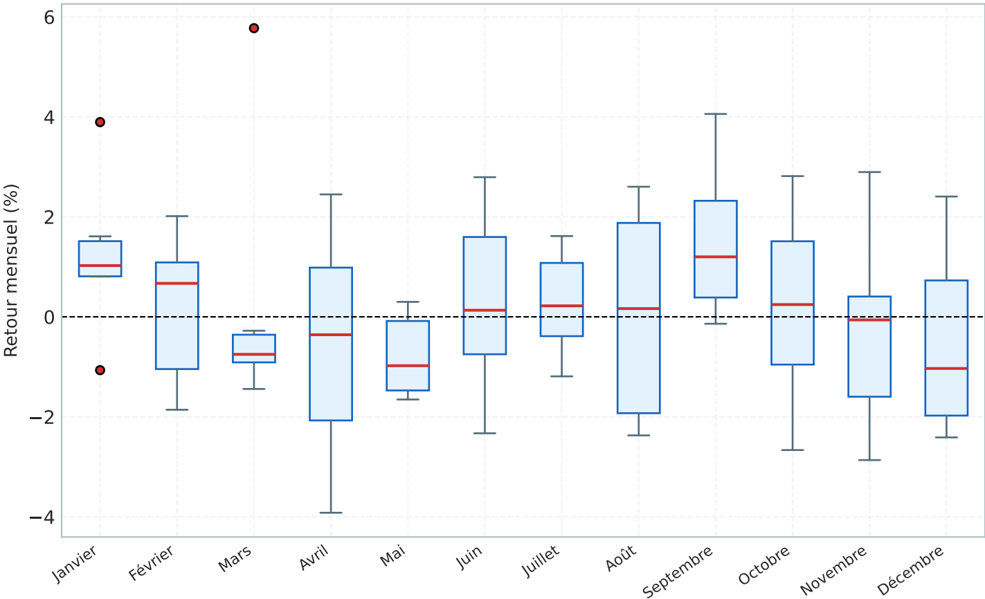
Graphique 3 : Distribution mensuelle des retours (%) pour USDCAD (2020-2025)
