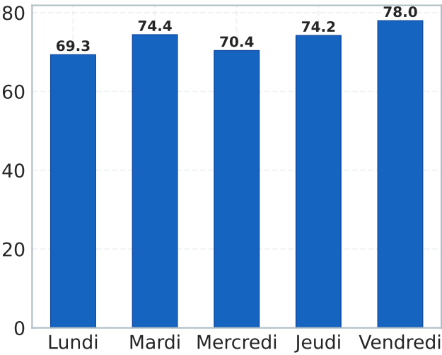
Amplitude moyenne par jour (Pips)
