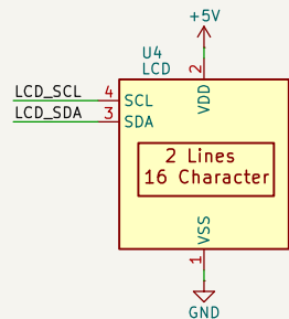
Display Module
