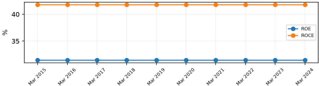
ROE / ROCE
