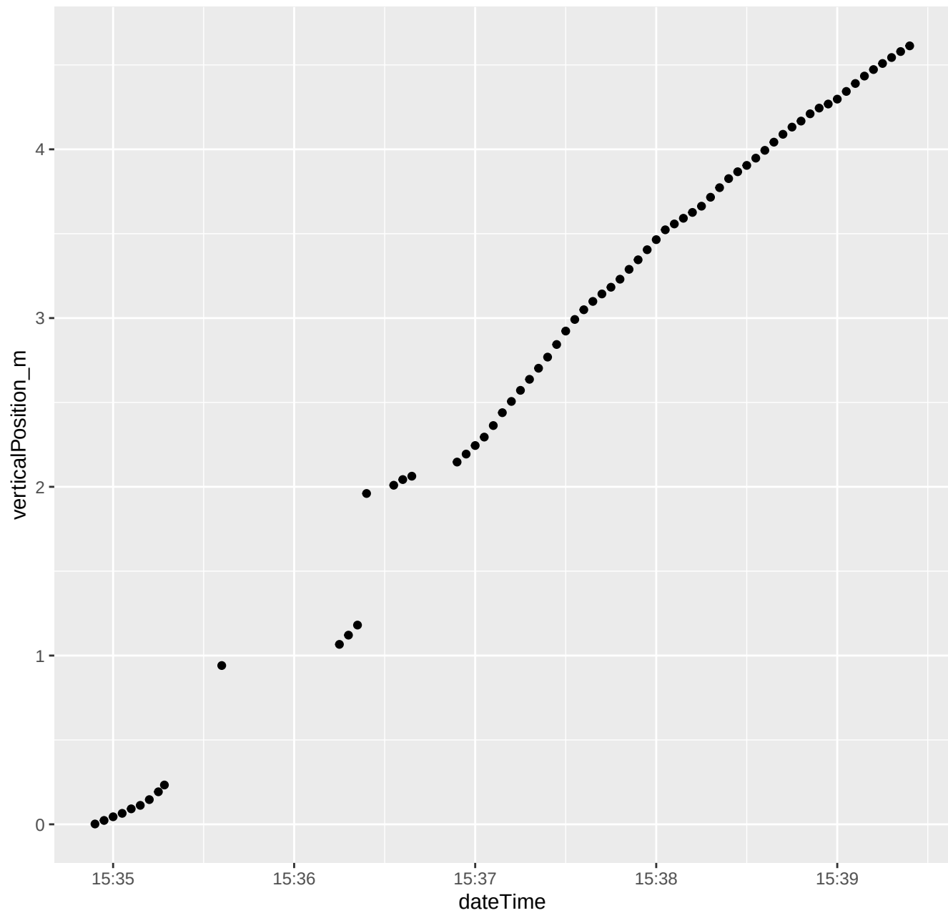
094_2017_08_08_Level1.csv ****Depth vs. time
