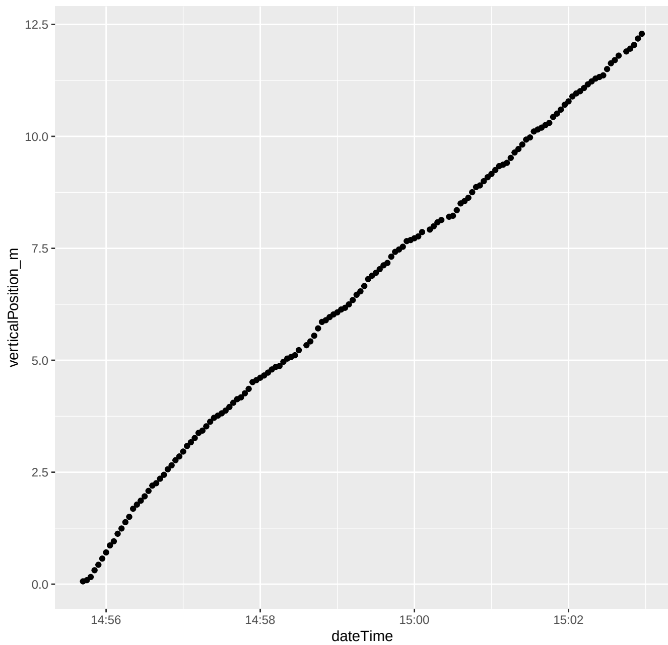
072_2024_08_20_Level1.csv ****Depth vs. time
