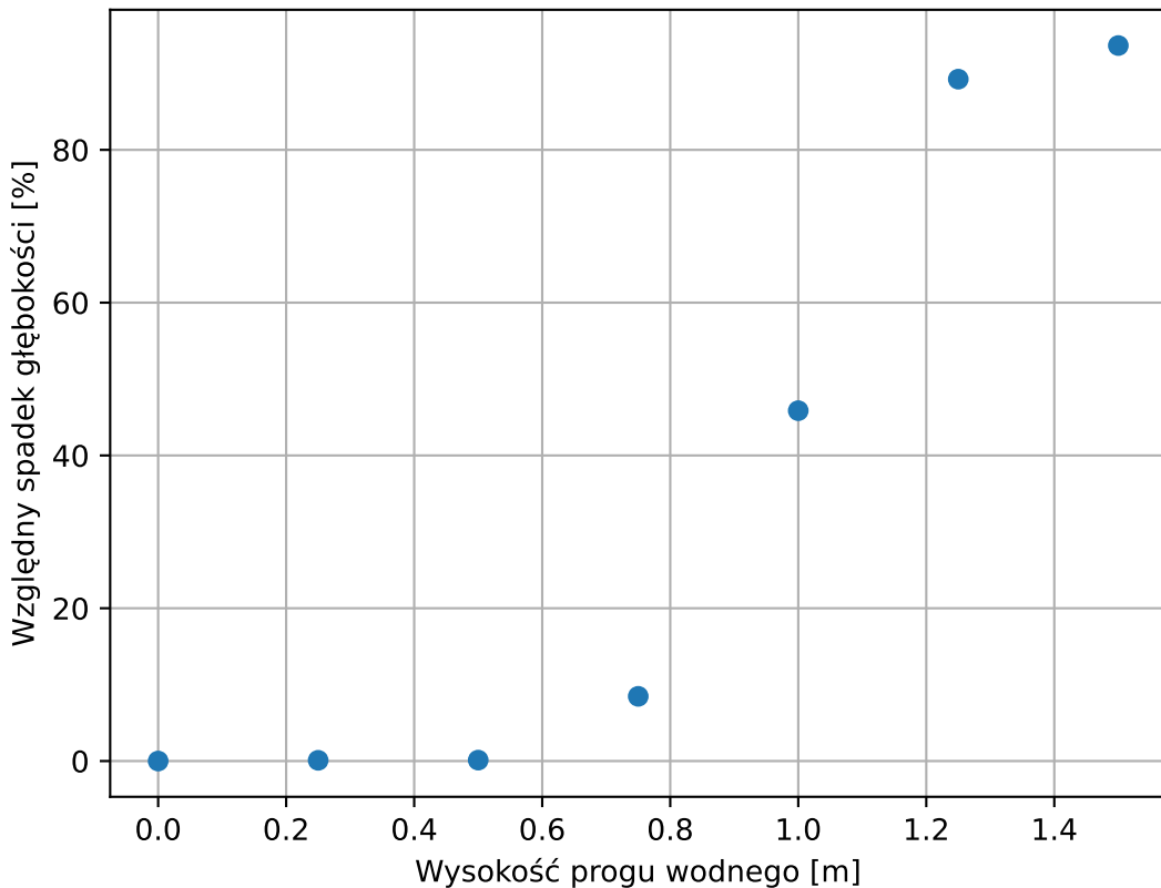
Zależność spadku głębokości wody od wysokości progu
