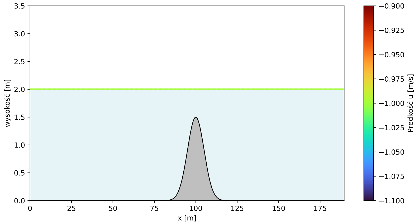
Rysunek 1. Wysokość oraz prędkość w chwili początkowej ( t=0s ) dla wysokości h=1.5m
