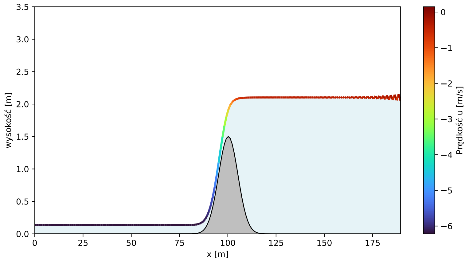
Rysunek 5. Wysokość oraz prędkość dla dwa razy większego \Delta t oraz \Delta x dla wysokości h=1.5\text{m} ( t=10000\text{s} )
