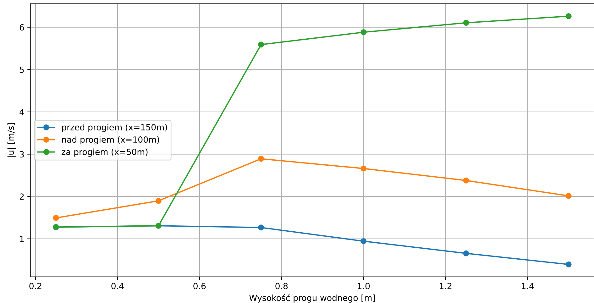
Rysunek 4. Zależność prędkości wody od wysokości progu (przed, na oraz za progiem)
