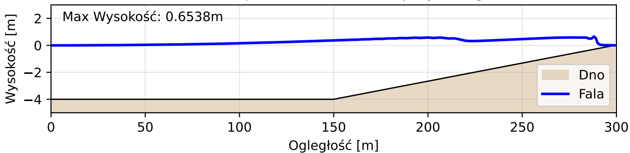
PRZEKRÓJ BOCZNY: Profil fali przy brzegu
