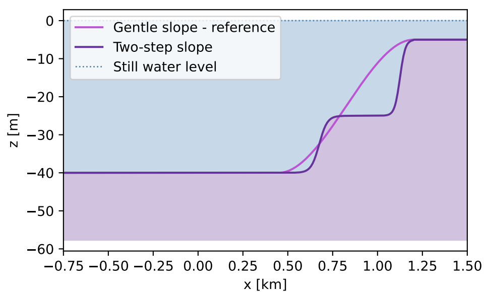
Rysunek 1. Rodzaje batymetrii przedstawione w pełnej długości domeny w x .
