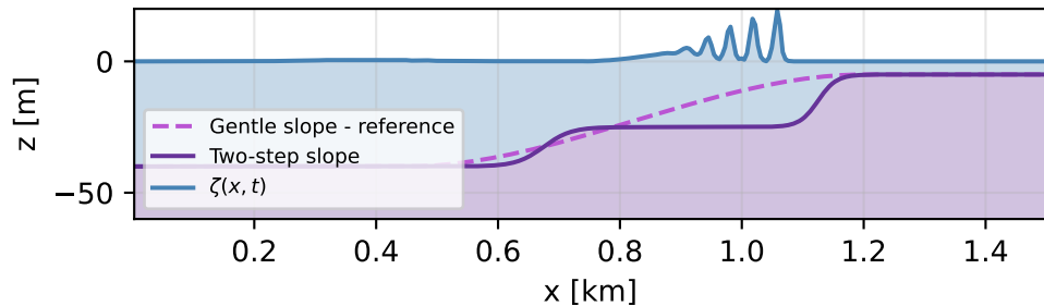
Rysunek 2. Klatka z animacji w przekroju.
