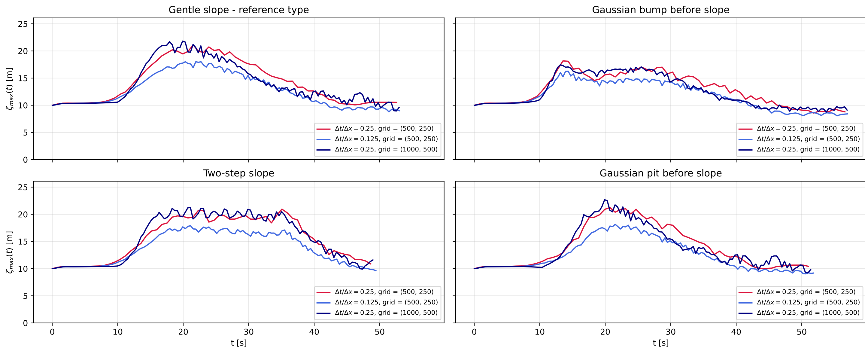
Rysunek 5. Maksymalne wysokości fali od momentu początku propagacji do dotarcia do brzegu dla różnych batymetrii i rozdzielczości siatek i czasu.
