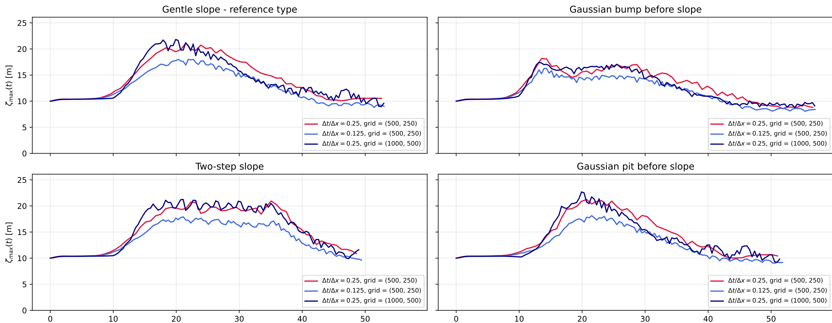
Rysunek 5. Maksymalne wysokości fali od momentu początku propagacji do dotarcia do brzegu dla różnych batymetrii i rozdzielczości siatek i czasu.
