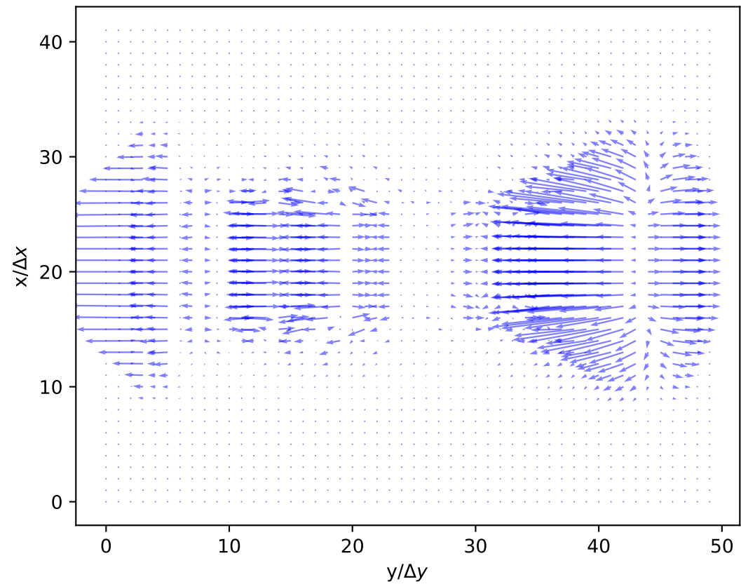
[v, u], siatka 500 \times 100
