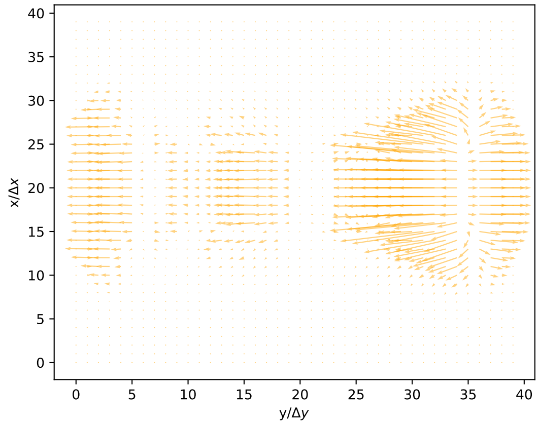
[v, u], siatka 1000 \times 200
