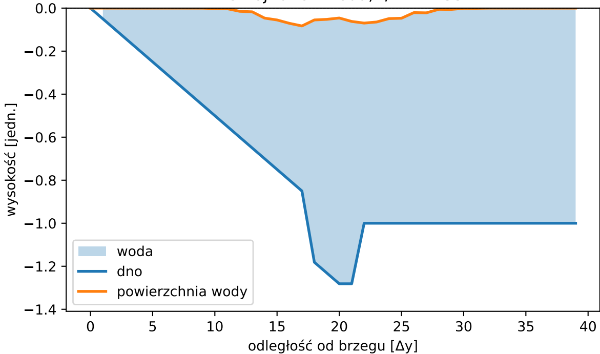
Przekrój: dno i woda, t/\Delta t = 135
