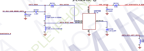
ANT3 FEED 天线3馈电
