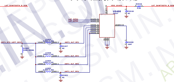
ANT1 E75 SP4T 天线1阻抗自动匹配
