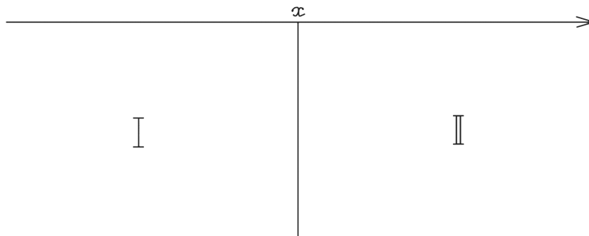
Рис. 4: Потенциальная дельта-яма
