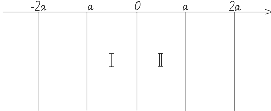
Рис. 7: Бесконечные дельта-ямы
