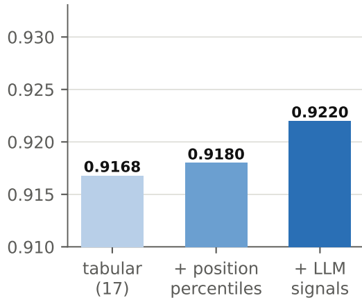
Row ROC-AUC
