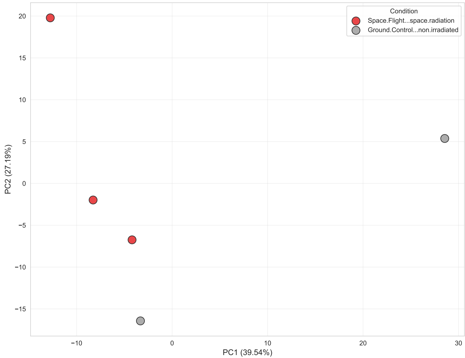
PCA - OSD-270
