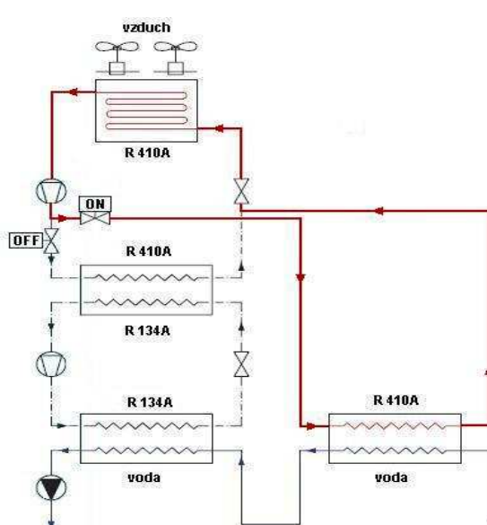
YUTAKI S80 při aktivaci jednoho okruhu
