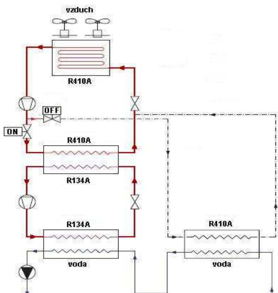
YUTAKI S80 při aktivaci dvou okruhů
