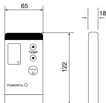
Drahtlose Fernbedienung
