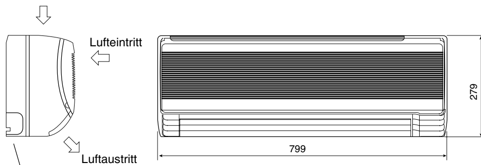
Frontansicht
