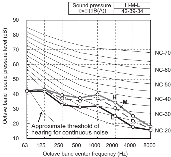
MMU-AP0074YH-E, AP0094YH-E, AP0124YH-E
