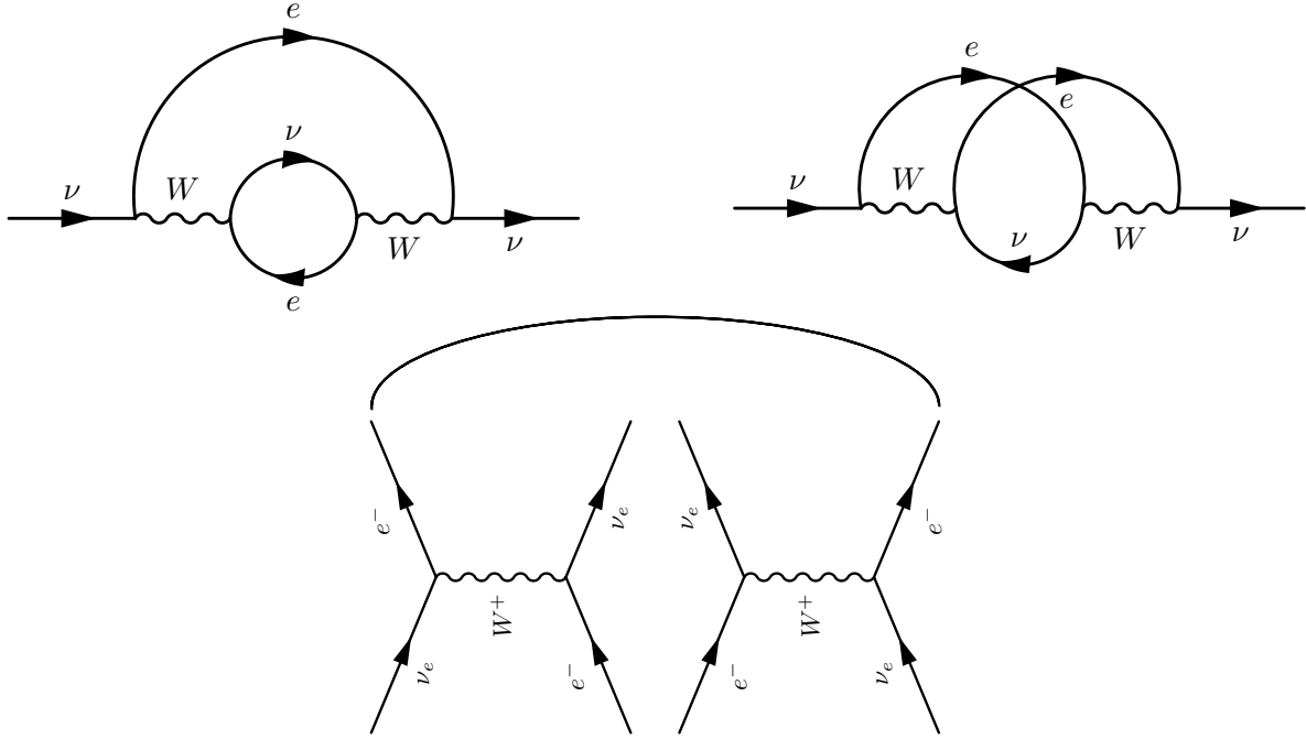
FIG. 3. ニュートリノ電子散乱の摂動2次の Feymann ダイアグラム。上2つがニュートリノが一旦別粒子へと変化した後にまたニュートリノへと戻るような確率過程としての衝突を示すダイアグラムである。下は摂動2次として、うまくニュートリノの外線だけを残すように2つの4点相互作用同士を繋ぐイメージを表している。
