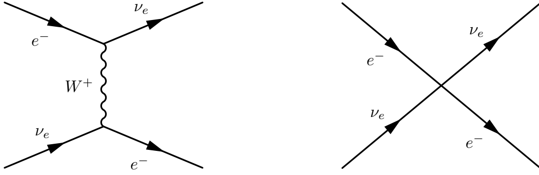
FIG. 1. ニュートリノ電子散乱の Feynman ダイアグラム。左は W ボソンあり、右は低エネルギー極限における 4 点相互作用に対応する。
