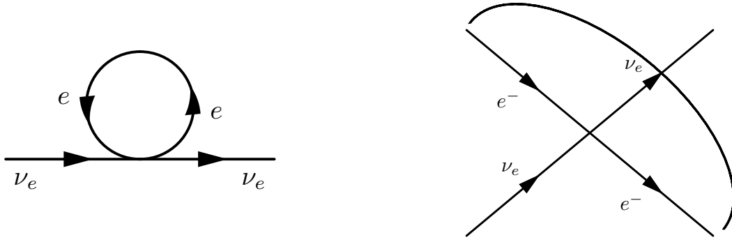
FIG. 2. ニュートリノ電子散乱の摂動1次の Feymann ダイアグラム。左が tadpole 型としてのポテンシャルで、右が元々の4点相互作用においてニュートリノ以外の背景物質の外線を繋いで丸めるイメージ図を表している。
