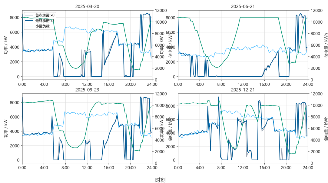
图 8 问题三四个指定日期的调度曲线
