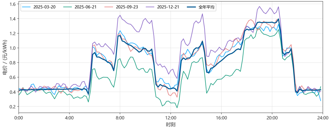
图 10 四个指定日期与全年平均的实时电价曲线
