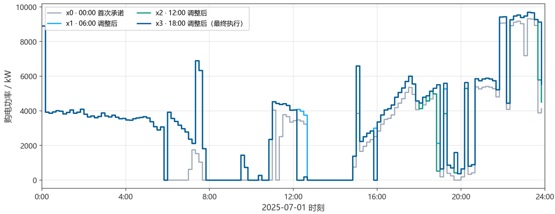
图 7 问题三某一日承诺路径的分阶段修订阶梯
