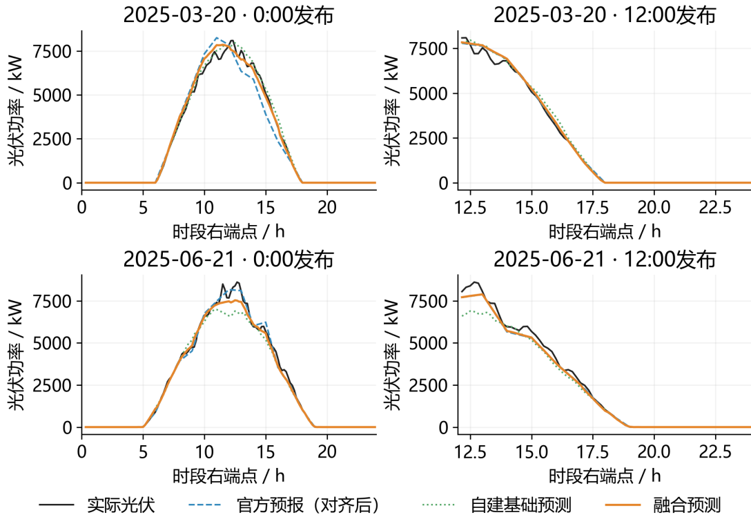
图 6 官方、自建与融合光伏预测的来源对照
