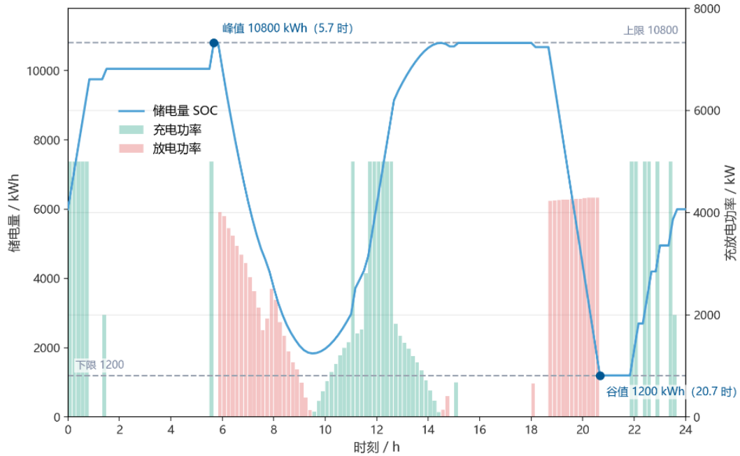
图 3 问题一储能 SOC 轨迹与充放电功率
