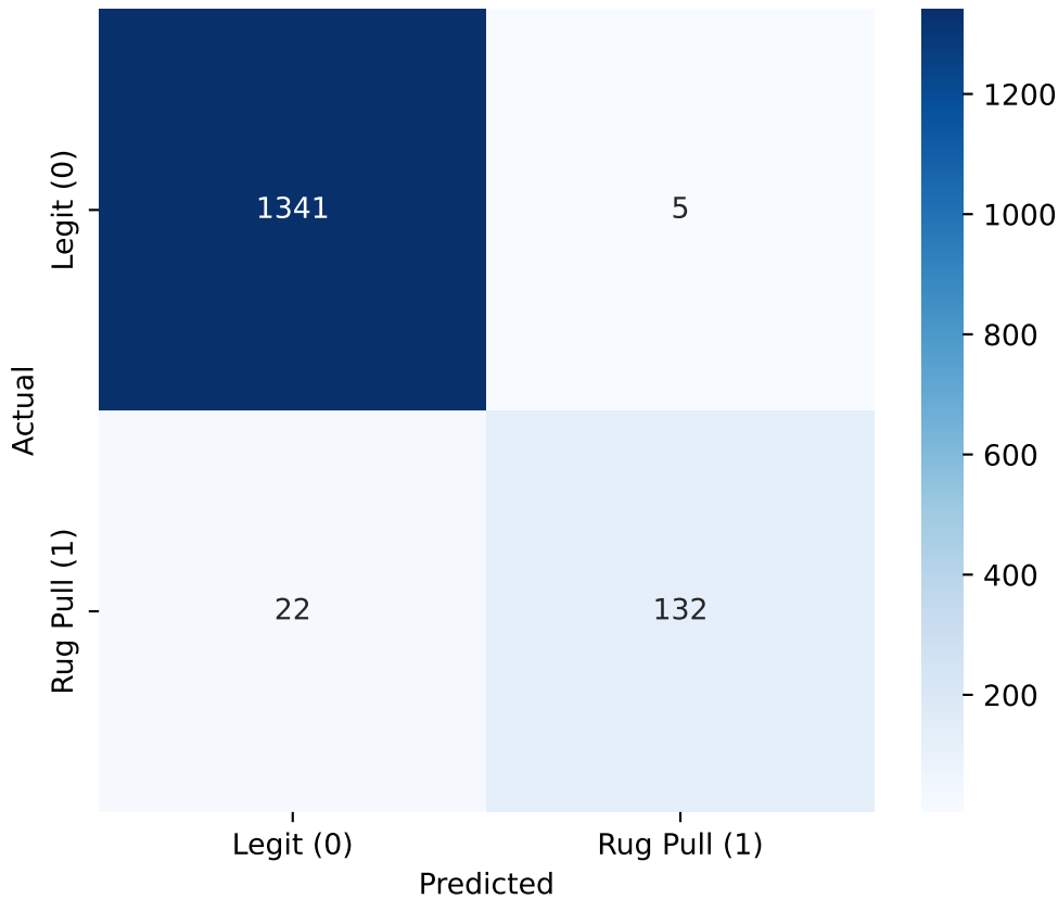
Confusion Matrix: Spatio-Temporal TGN
