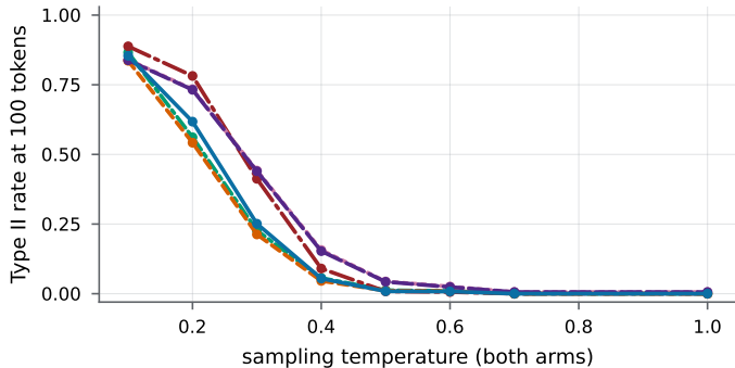
OPT-1.3B
