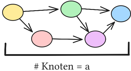
Abhängigkeits-Graph
