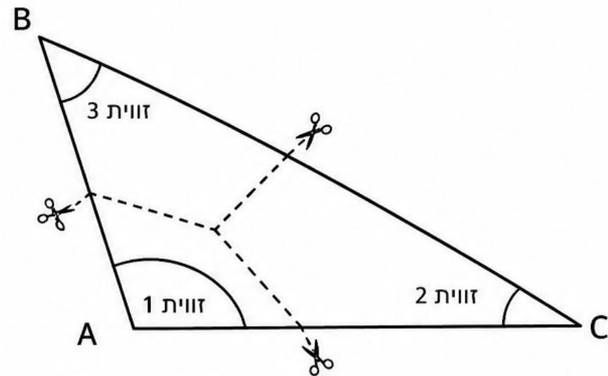
משולש קהה זווית
