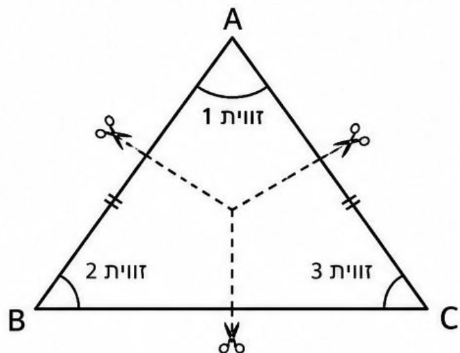
משולש שווה צלעות
