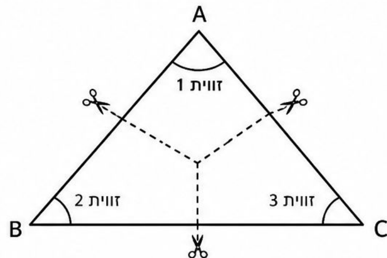
משולש חד זווית
