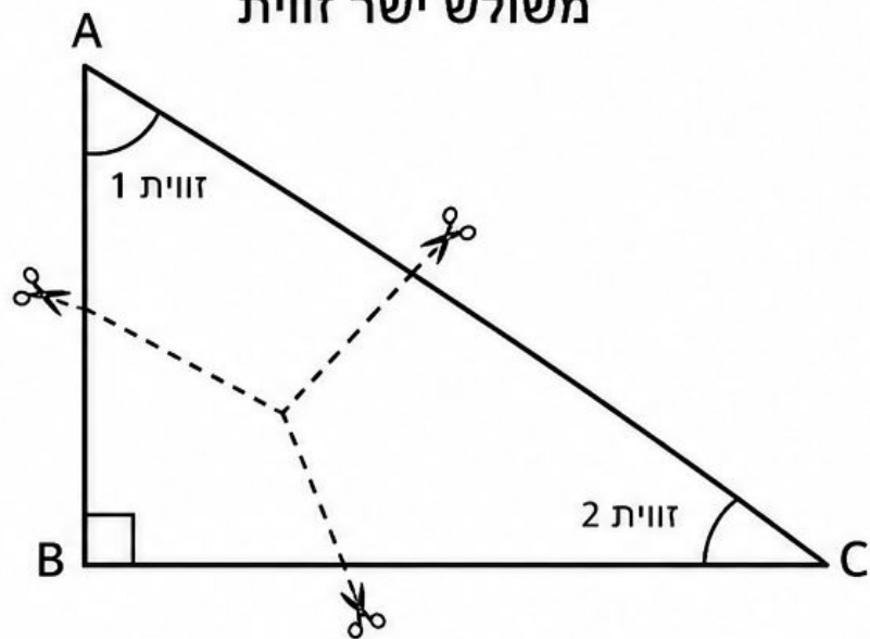
משולש ישר זווית
