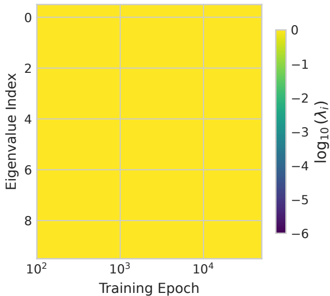
Mlp
