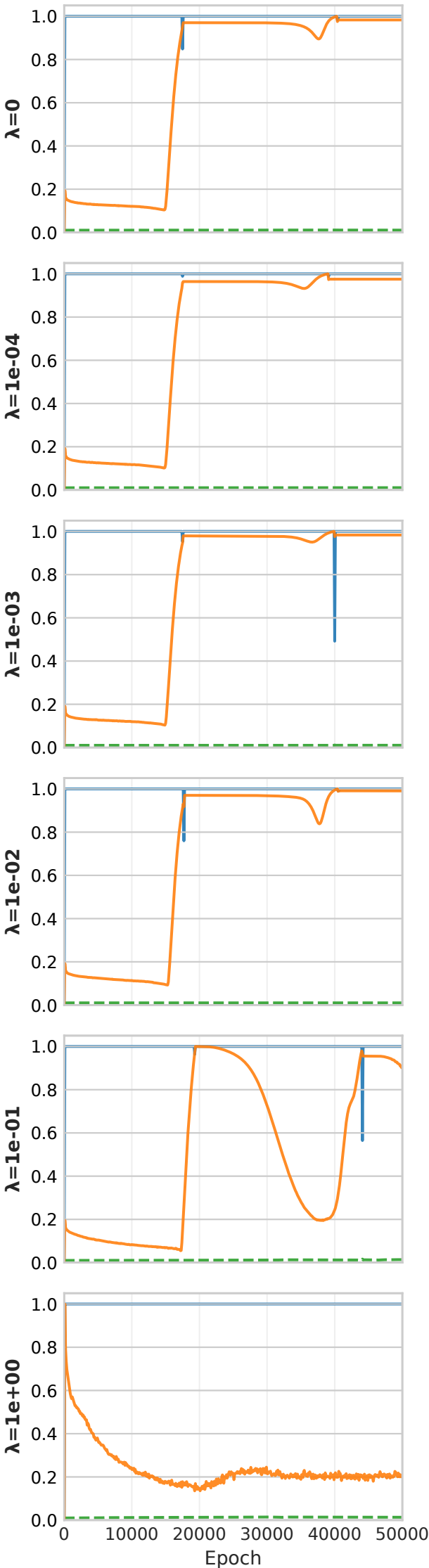
ADAMW
