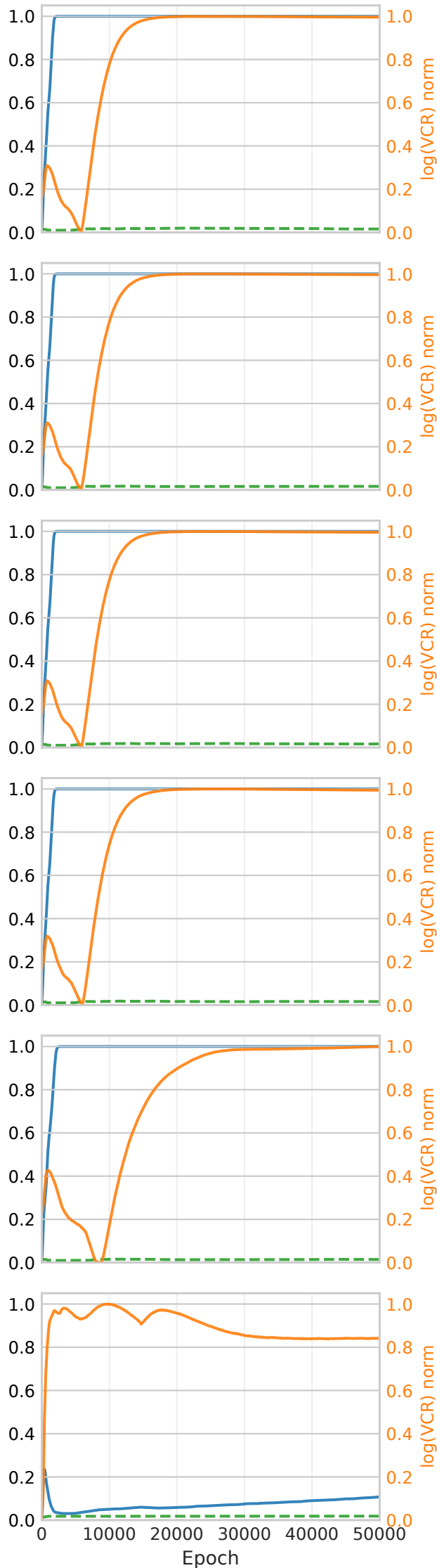
MUON
