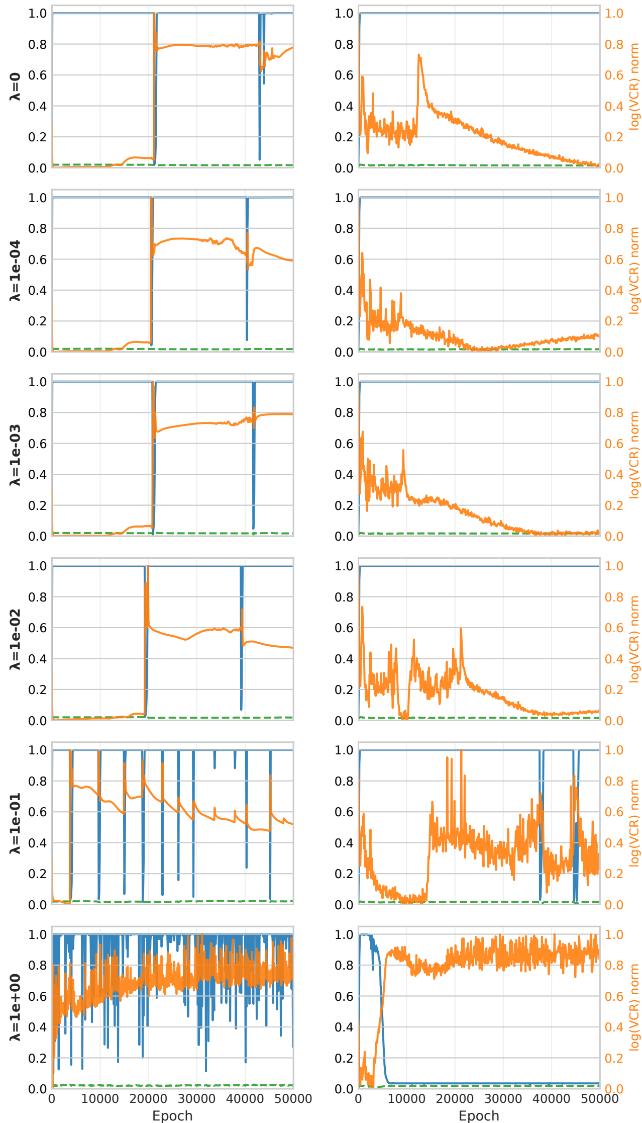
ADAMW
