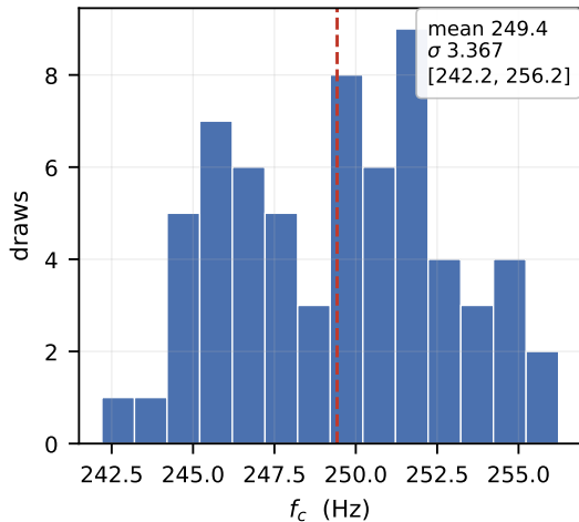
(a) scale: \sigma = 3.367 Hz (1.35 %)
