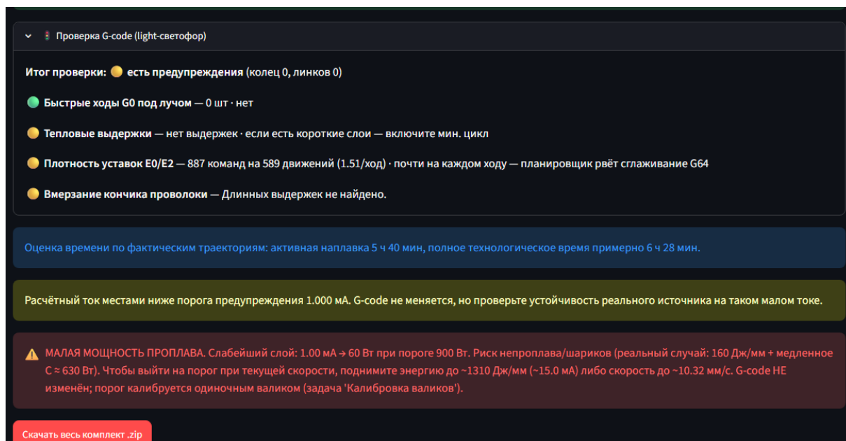
Рисунок 6 — Пример блока автоматической проверки готового G-code
