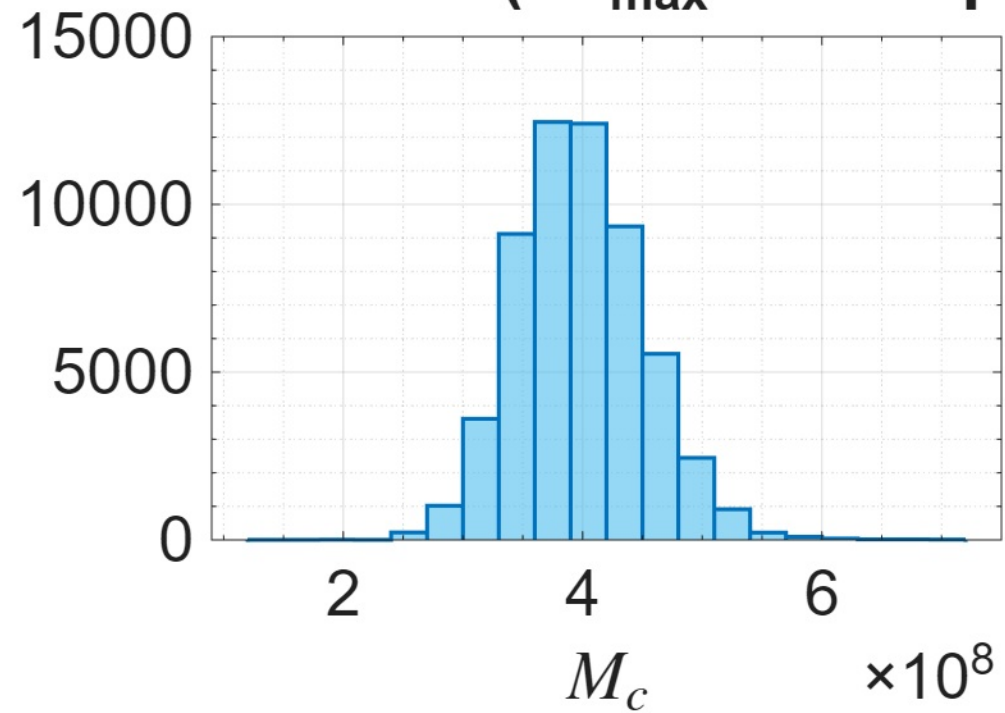
UGC02455 ( R_{\text{max}} = 4.03\text{kpc} )
