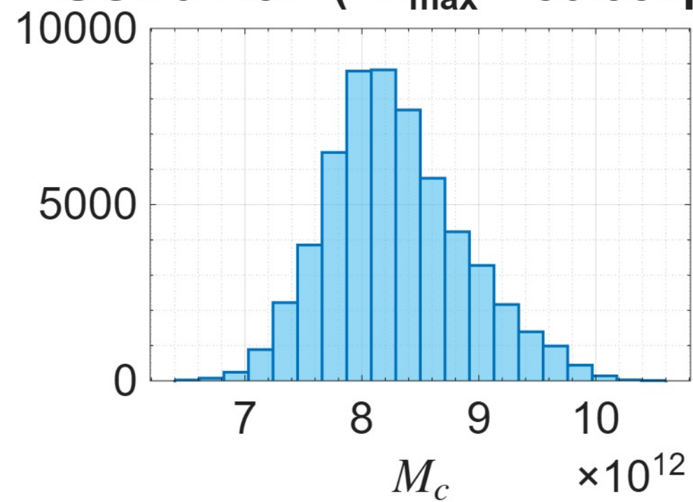
UGC02487 ( R_{\text{max}} = 80.38\text{kpc} )
