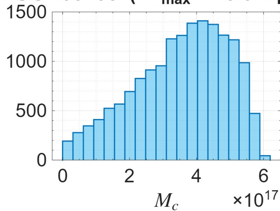
UGC03205 ( R_{\text{max}} = 40.04\text{kpc} )
