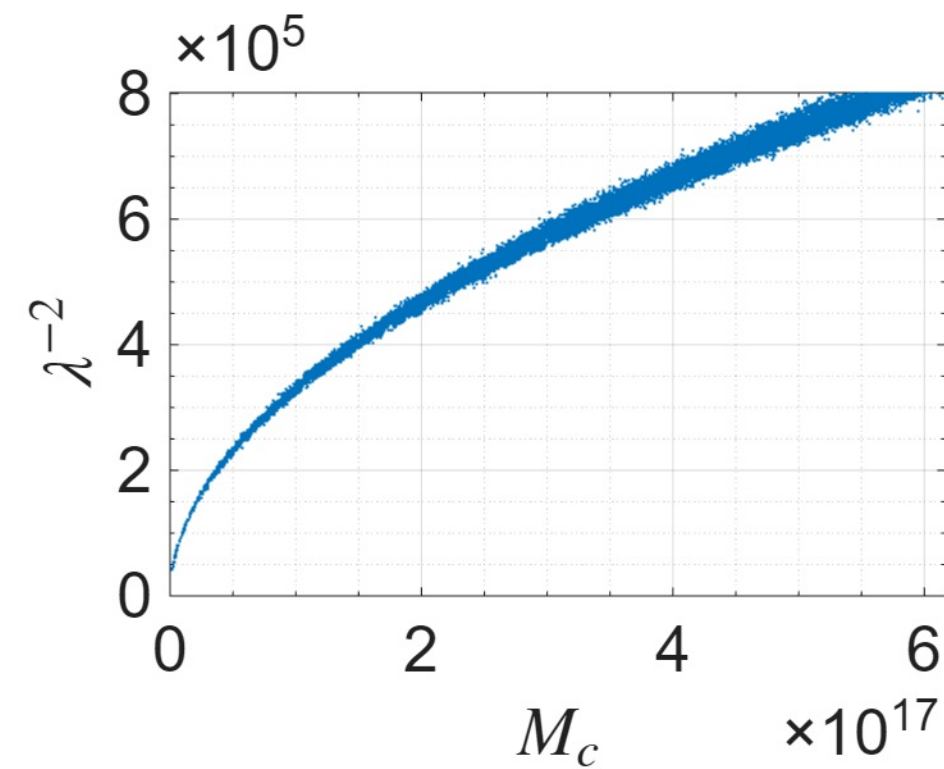
UGC03205 ( R_{\text{max}} = 40.04\text{kpc} )
