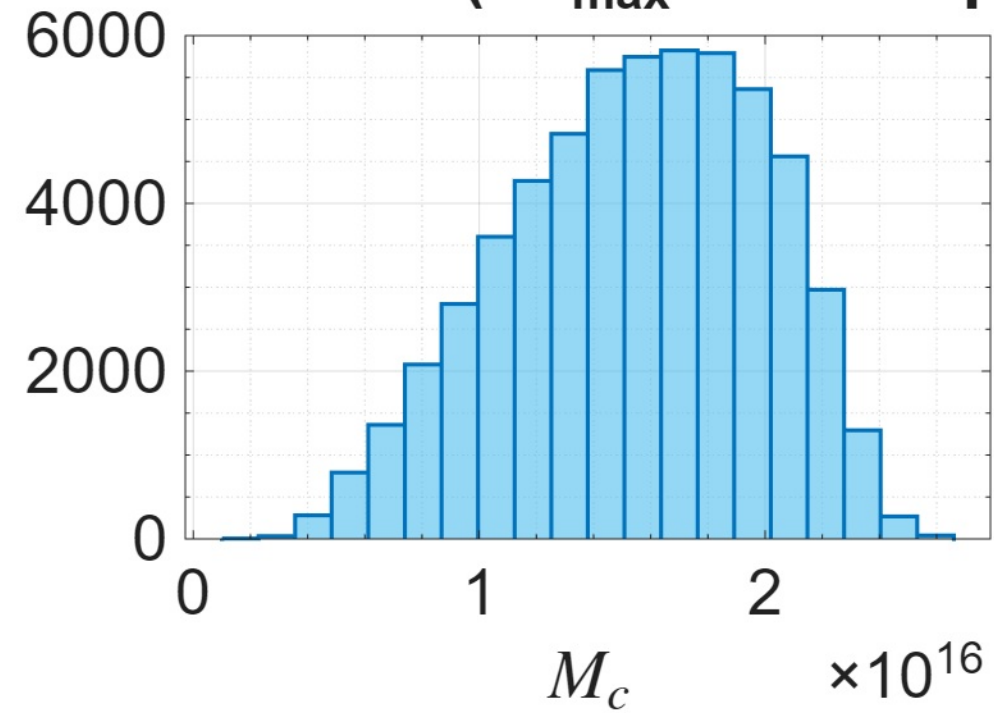
UGC03546 ( R_{\text{max}} = 29.23\text{kpc} )
