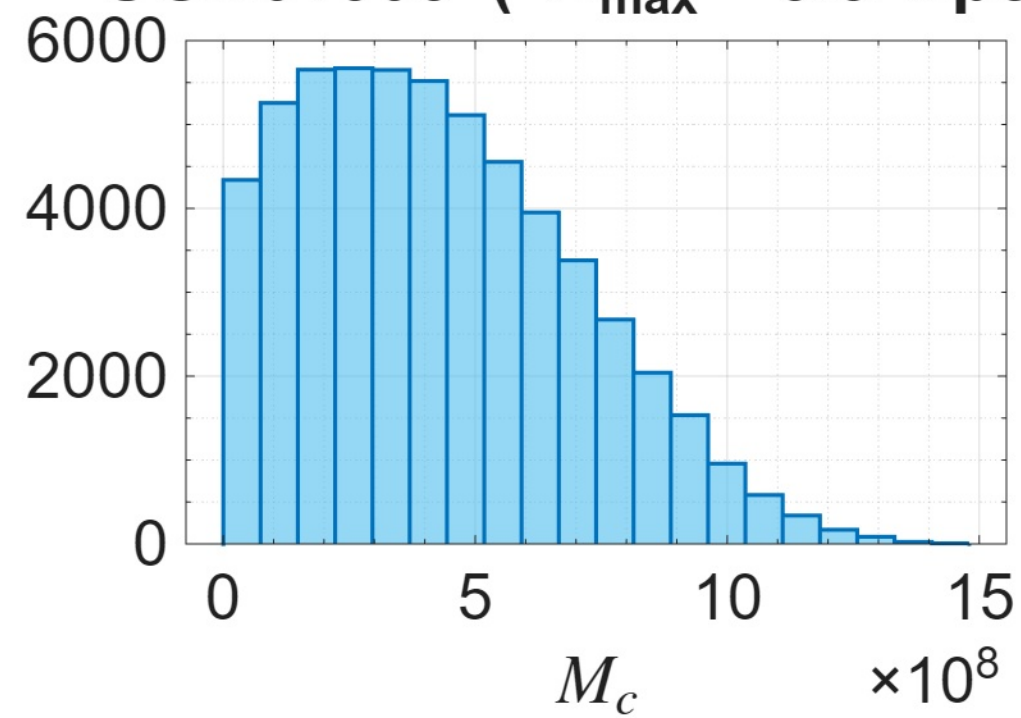
UGC04305 ( R_{\text{max}} = 5.52\text{kpc} )
