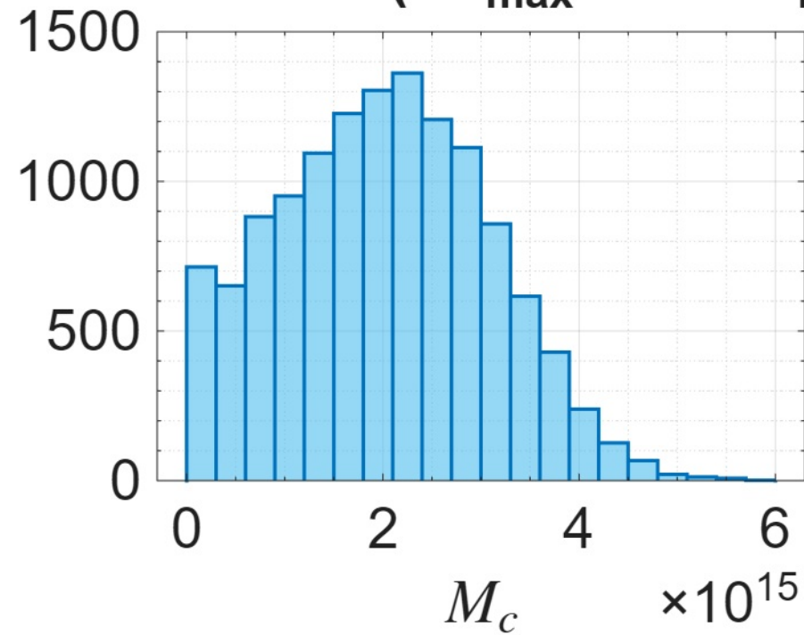
UGC05414 ( R_{\text{max}} = 4.11\text{kpc} )
