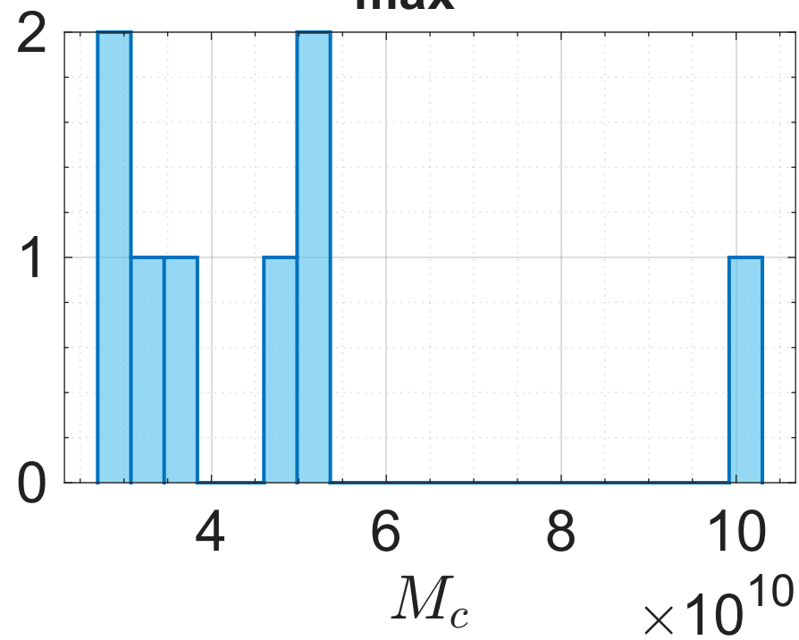
IC2574 ( R_{\text{max}}=10.23\text{kpc} )
