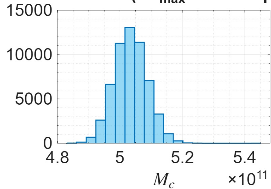
UGC00128 ( R_{\text{max}} = 53.75\text{kpc} )
