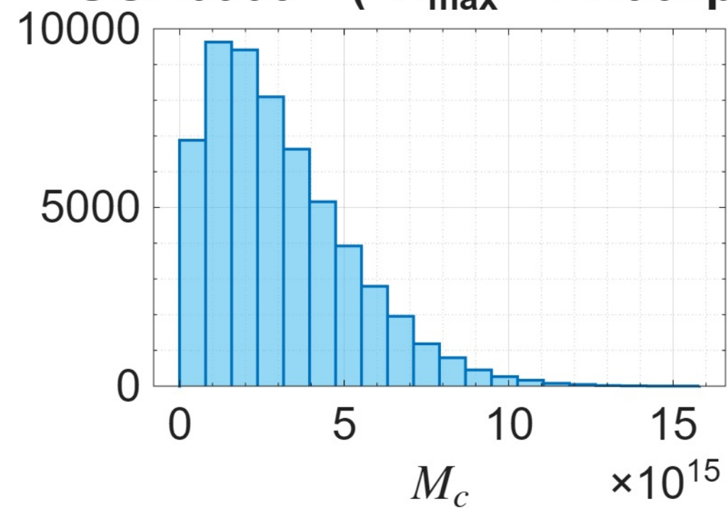
UGC09037 ( R_{\text{max}} = 27.96\text{kpc} )
