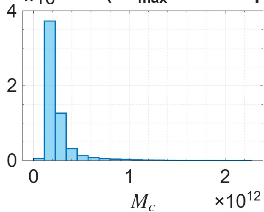
UGC05999 ( R_{\text{max}} = 16.22\text{kpc} )
