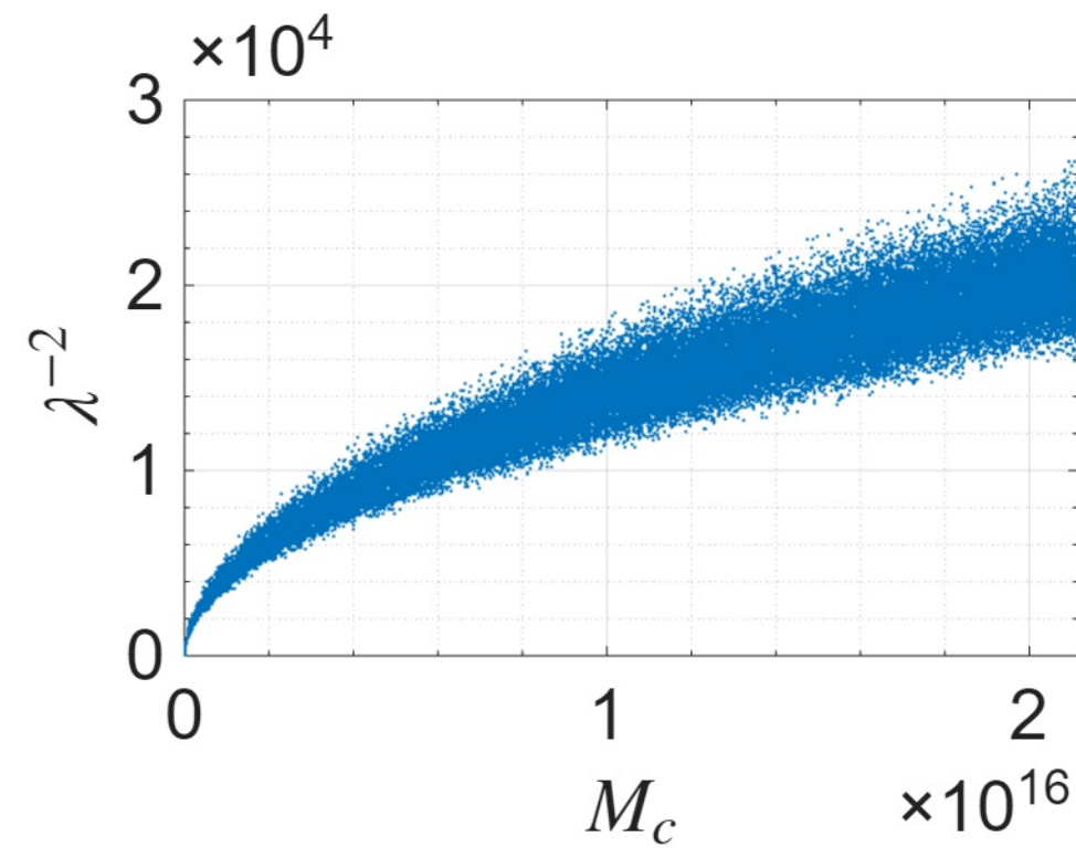
UGC06399 ( R_{\text{max}} = 7.85\text{kpc} )
