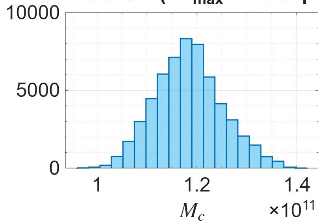
UGC06667 ( R_{\text{max}} = 7.85\text{kpc} )
