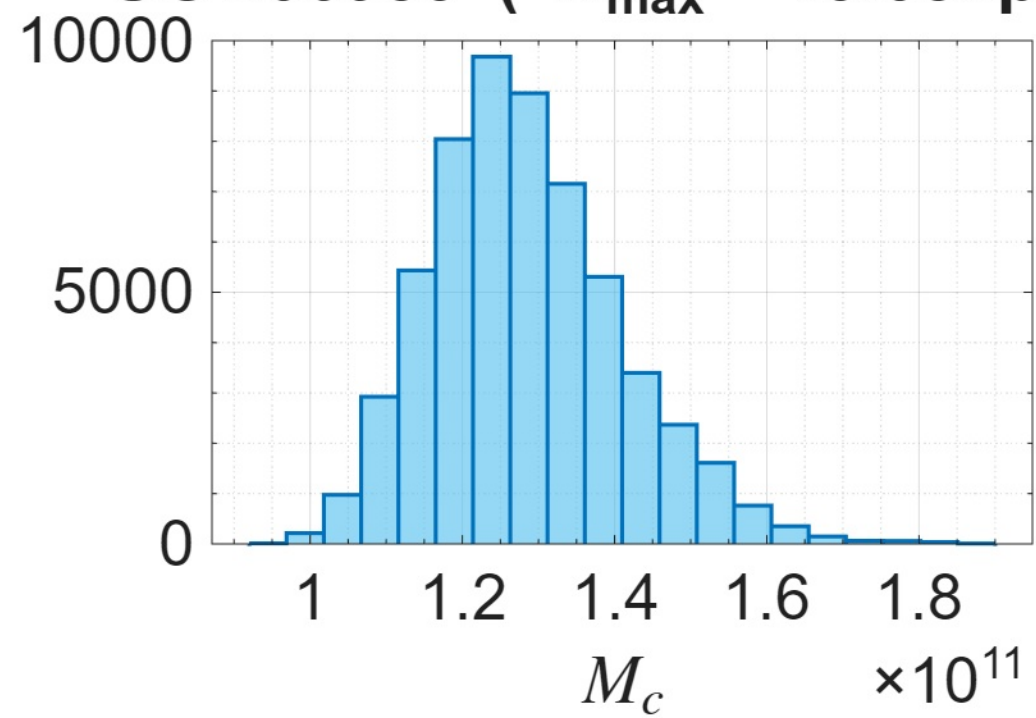
UGC06983 ( R_{\text{max}} = 15.68\text{kpc} )
