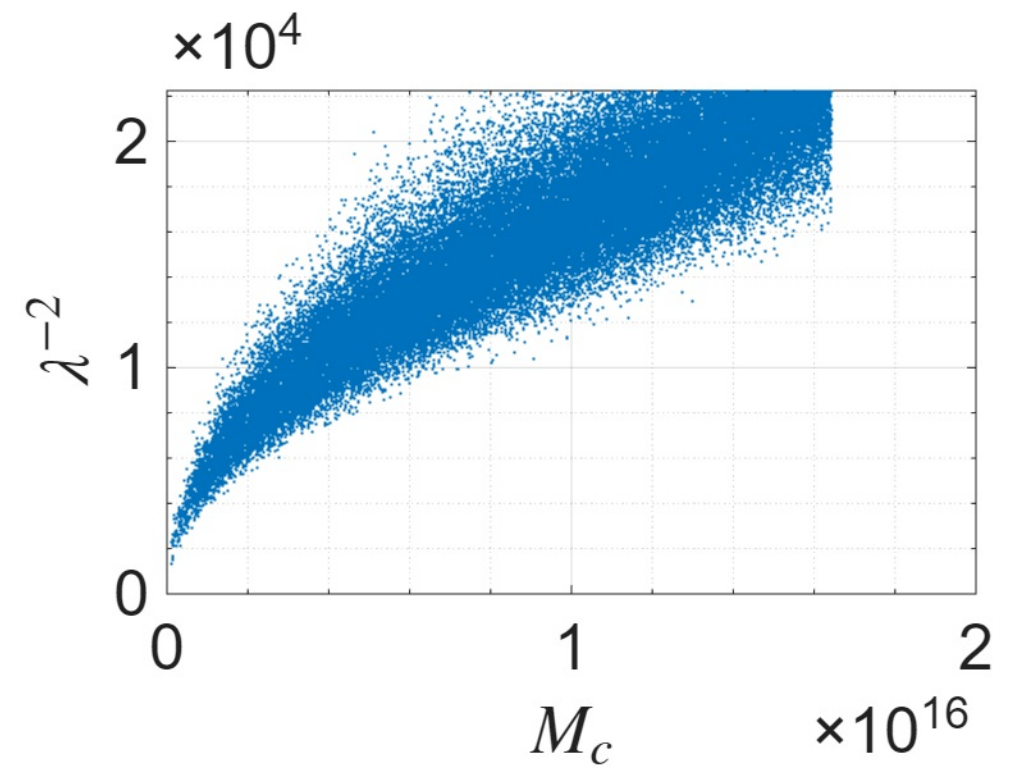
UGC07261 ( R_{\text{max}} = 6.67\text{kpc} )
