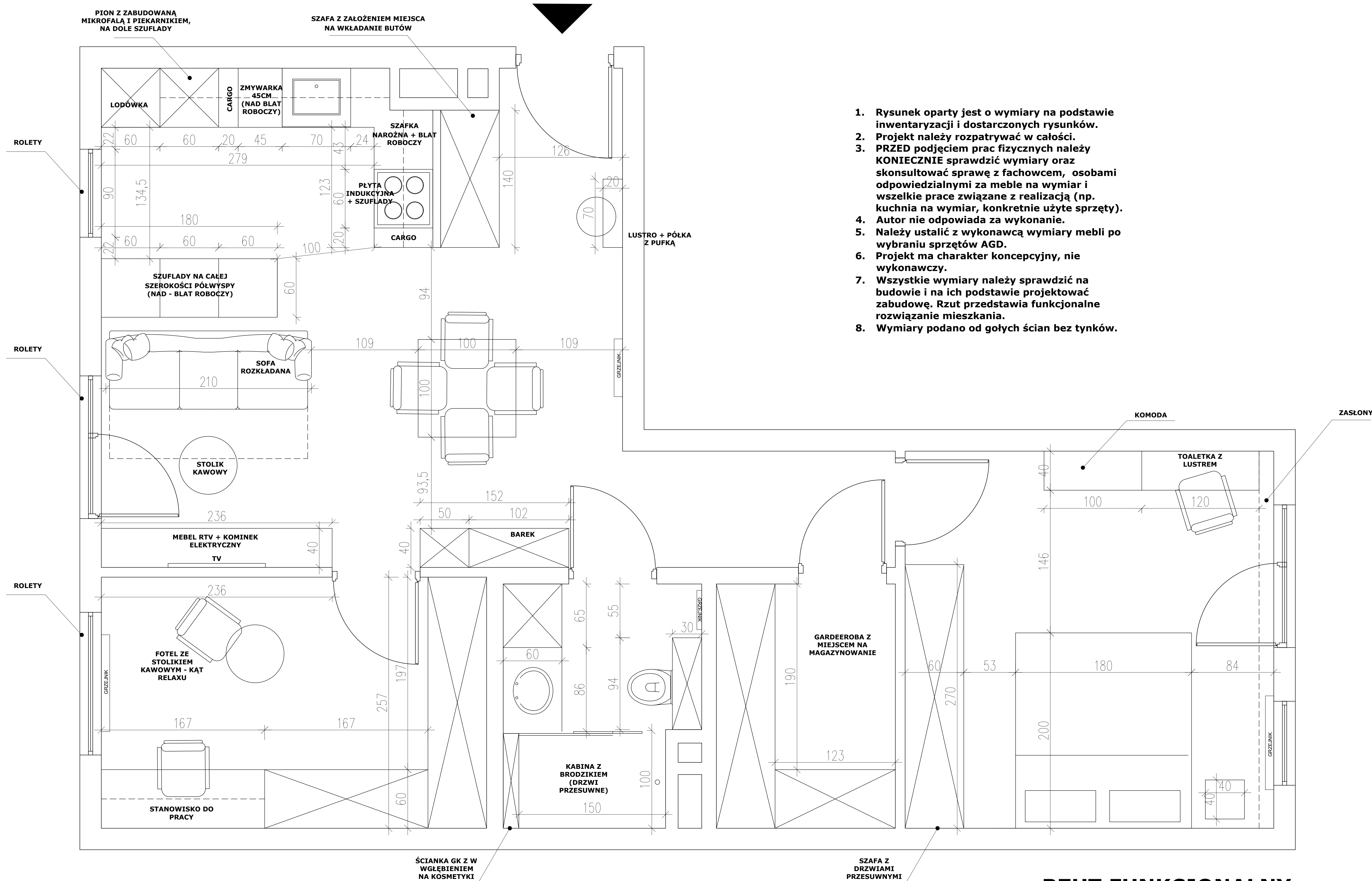
RZUT FUNKCJONALNY
